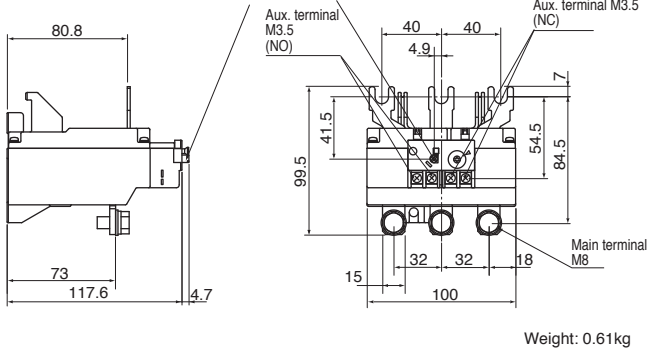
3NK4F*
