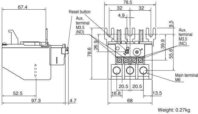
3NK4F*
