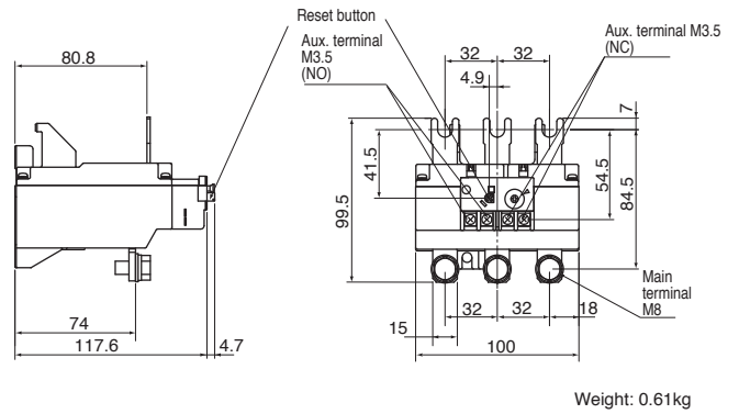
3NK4Q*
