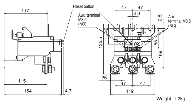
3NK4Q*
